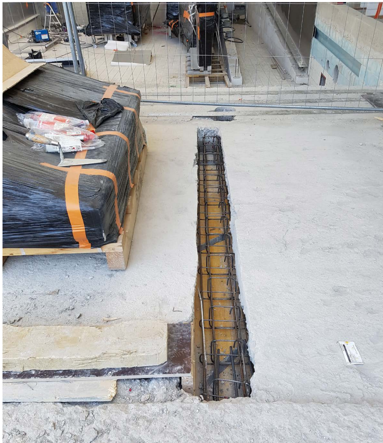
Consolidation de la structure des plages des bassins, avec la mise en place de poutres en béton armé.
