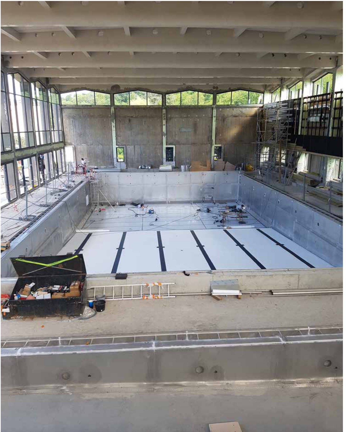
Vue d'ensemble du grand bassin avec son revêtement posé.
