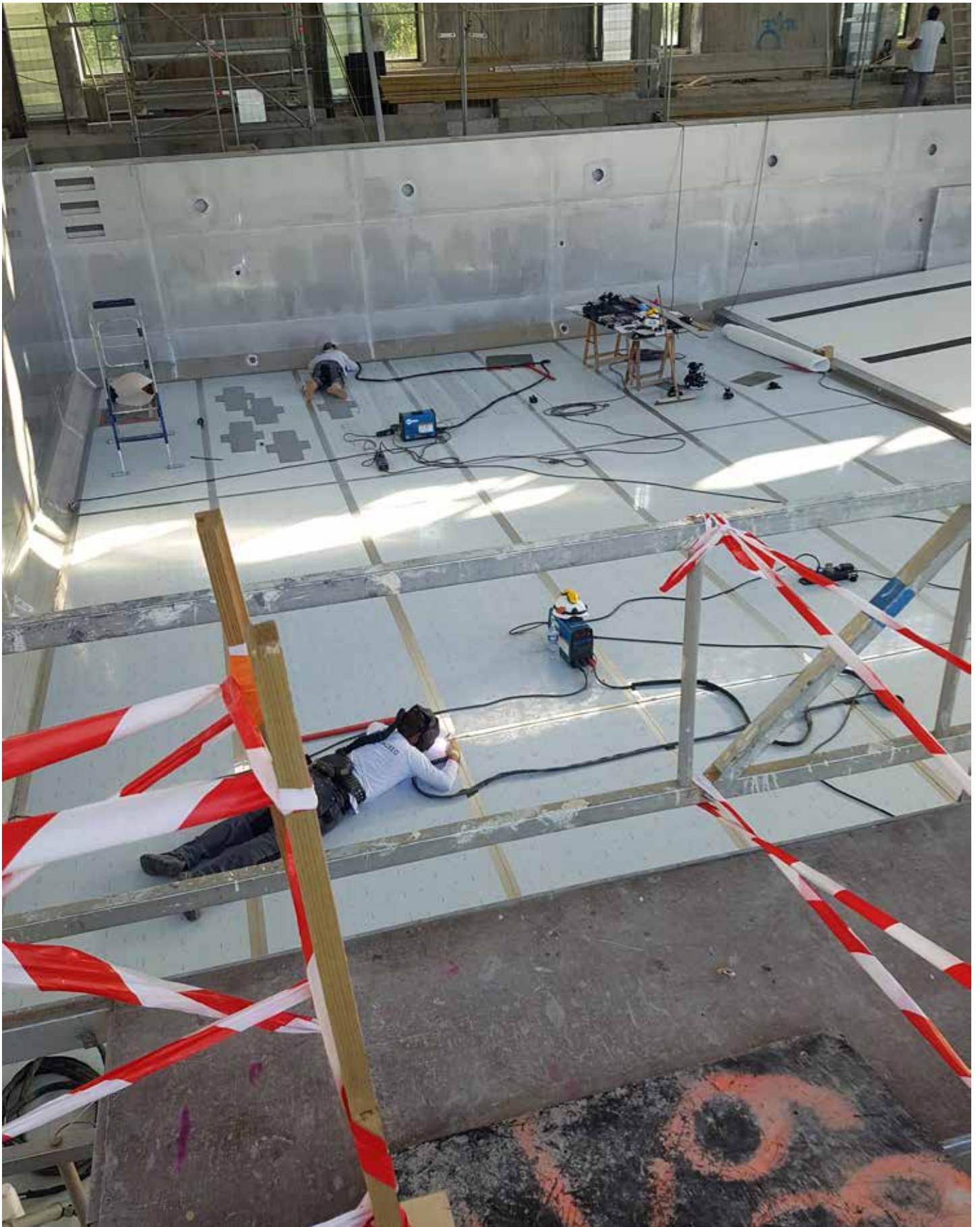
Soudure des plaques d'inox sur le fond du grand bassin par les techniciens.
