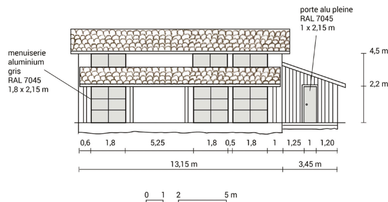
FAÇADE SUD
